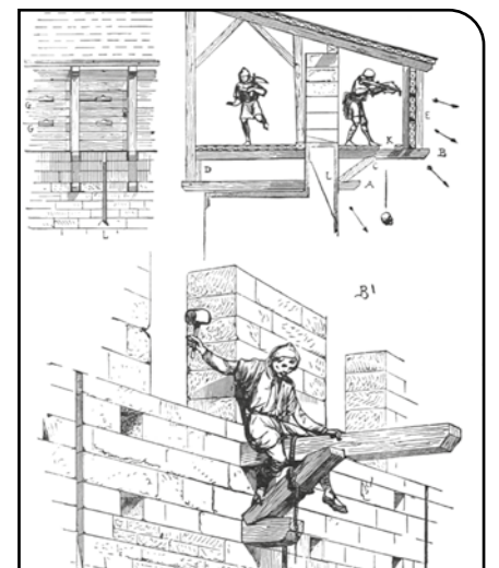
Dessin d'un hourd fixé sur le rempart Viollet-le-Duc - Dessin extrait de l'ouvrage La cité de Carcassonne : Figure N°13
